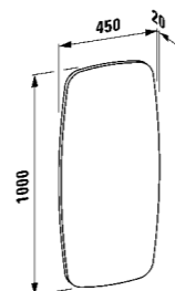
44255.5.055.000.1 Mirror without lighting Spiegel ohne Beleuchtung Miroir sans éclairage Specchio senza illuminazione
