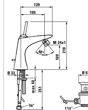
3.1155.1.004.110.1 Basin single-lever mixer, without pop-up, with joystick cartridge and fixed spout, spout reach 105 mm Waschtischmischer ohne Ablaufventil, mit Joystick-Patrone und festem Auslauf, Ausladung 105 mm Mitigeur de lavabo, sans vidage, avec cartouche joystick et goulot fixe, saillie 105 mm Miscelatore lavabo senza piletta, con cartuccia joystick e bocca di erogazione fissa, sporgenza 105 mm
