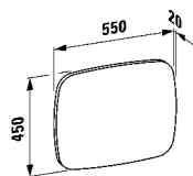
44155.5.055.000.1 Mirror without lighting Spiegel ohne Beleuchtung Miroir sans éclairage Specchio senza illuminazione
