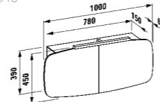
44455.5 Mirror cabinet with lighting, 1 lighting element 230V/8W IP44, 2 coupled mirror doors, glass shelf, no switch, no socket Spiegelschrank mit Beleuchtung, 1 Beleuchtungselement 230V/8W IP44, 2 Doppelspiegeltüren, Glasfachboden, kein Schalter, keine Steckdose Armoire de toilette à miroir avec éclairage, 1 élément d'éclairage 230V/8W IP44, 2 portes à miroir double, étagère en verre, sans interrupteur, sans prise Armadietto a specchio con illuminazione, 1 lampada 230V/8W IP44, 2 ante a specchio doppio, ripiano in vetro, senza interruttore, senza presa
