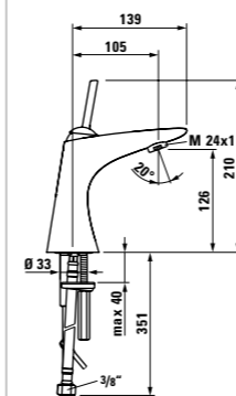
3.1155.1.004.110.1 Basin single-lever mixer, without pop-up, with joystick cartridge and fixed spout, spout reach 105 mm Waschtischmischer ohne Ablaufventil, mit Joystick-Patrone und festem Auslauf, Ausladung 105 mm Mitigeur de lavabo, sans vidage, avec cartouche joystick et goulot fixe, saillie 105 mm Miscelatore lavabo senza piletta, con cartuccia joystick e bocca di erogazione fissa, sporgenza 105 mm
