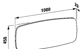
44255.5.055.000.1 Mirror without lighting Spiegel ohne Beleuchtung Miroir sans éclairage Specchio senza illuminazione
