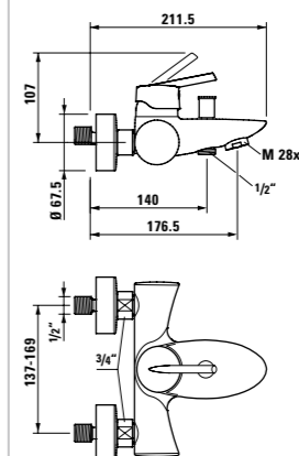
3.1155.1.004.110.1 Basin single-lever mixer, without pop-up, with joystick cartridge and fixed spout, spout reach 105 mm Waschtischmischer ohne Ablaufventil, mit Joystick-Patrone und festem Auslauf, Ausladung 105 mm Mitigeur de lavabo, sans vidage, avec cartouche joystick et goulot fixe, saillie 105 mm Miscelatore lavabo senza piletta, con cartuccia joystick e bocca di erogazione fissa, sporgenza 105 mm
