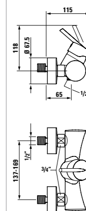
3.3155.7.004.145.1 Shower single-lever mixer complete, with Ecototal cartridge, Comfort Tre handspray and flexible hose 1800 mm Duschenmischer komplett, mit Ecototal-Patrone, Comfort Tre Handbrause und Kunststoffschlauch 1800 mm Mitigeur de douche complet, avec cartouche Ecototal, douchette Comfort Tre et flexible synthétique 1800 mm Miscelatore doccia completo, con cartuccia Ecototal, doccetta Comfort Tre e tubo sintetico 1800 mm
