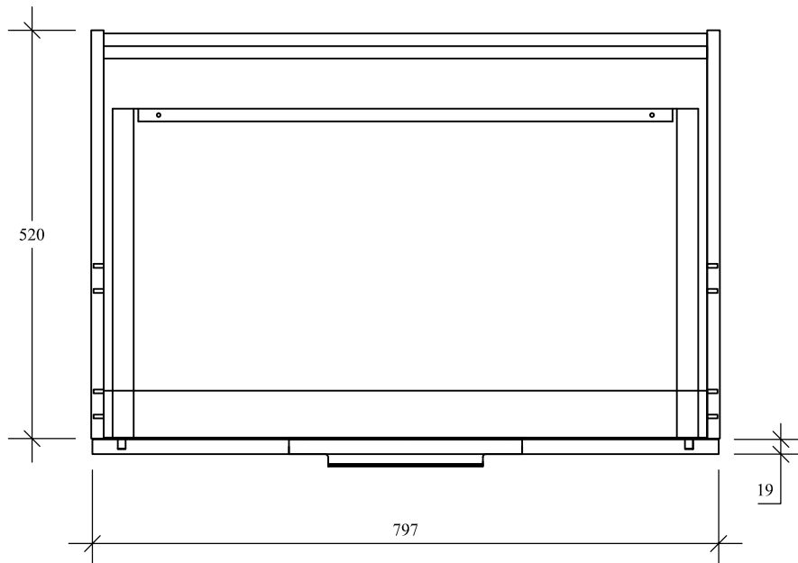
Draufsicht
