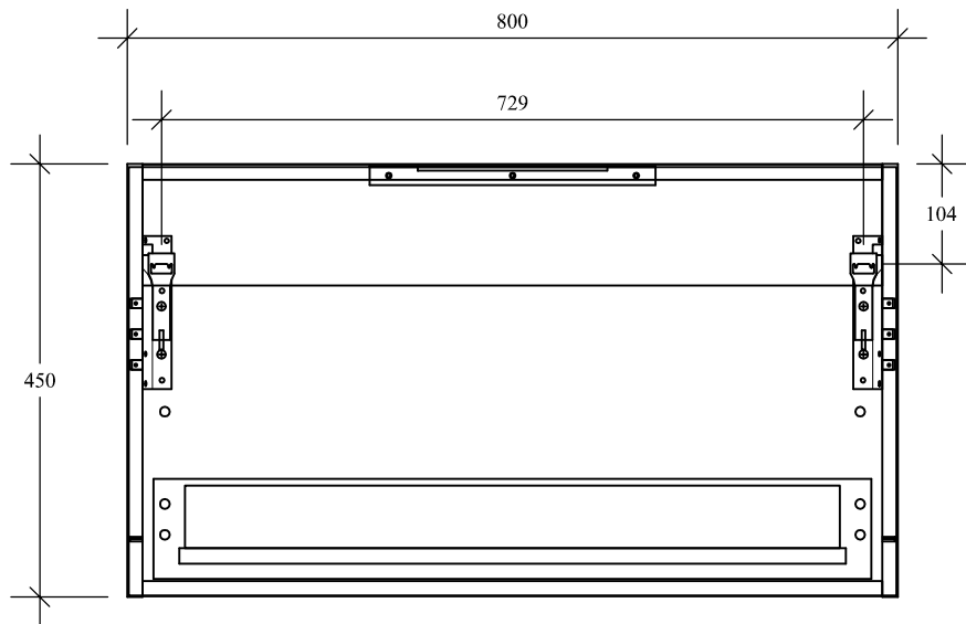
Draufsicht
